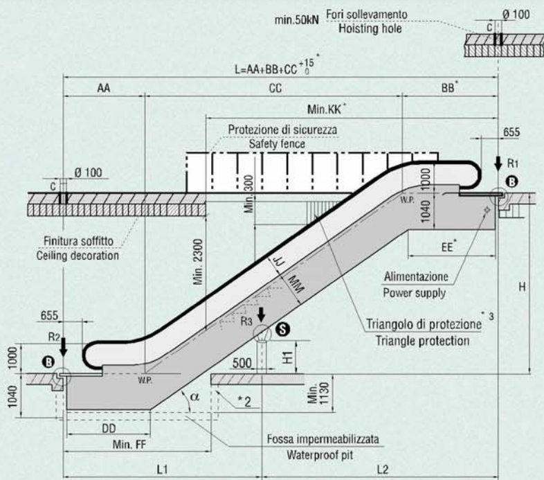
Apertura superiore/Upper floor opening Min. KK
