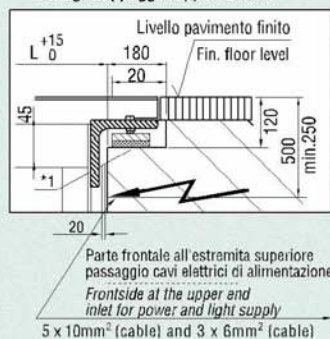
Particolare/Detail B Dettaglio appoggi/Support access
